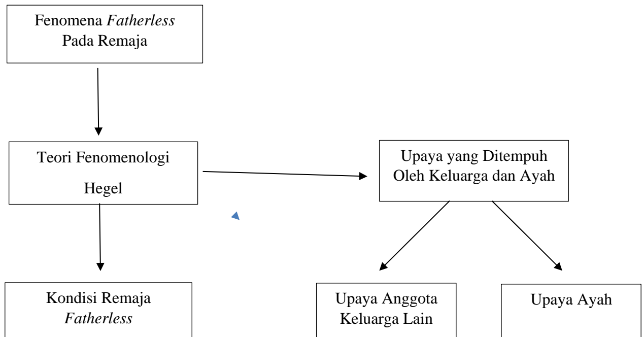
Gambar 2.6 Kerangka Teori
