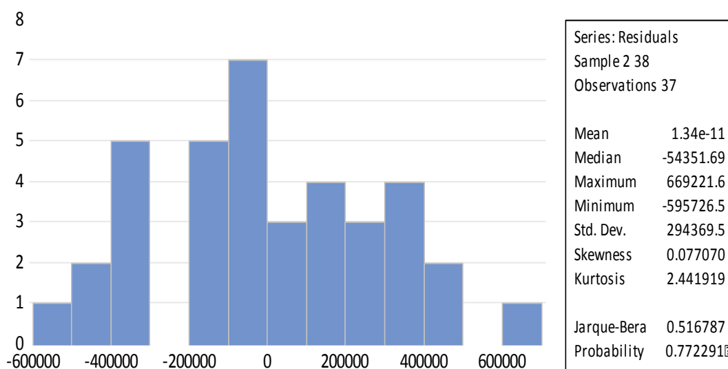
Grafik 4.1 Histogram
